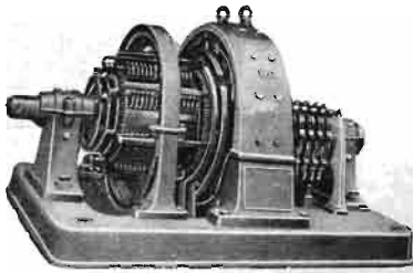
зад, покретана мотором са стране, може да даје истовремено једносмислену и наизменичну струју. (На сл.: 1. комутатор, 2. комутаторка веће снаге).
