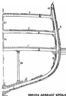
ПРЕСЕК ДРВЕНОГ БРОДА
