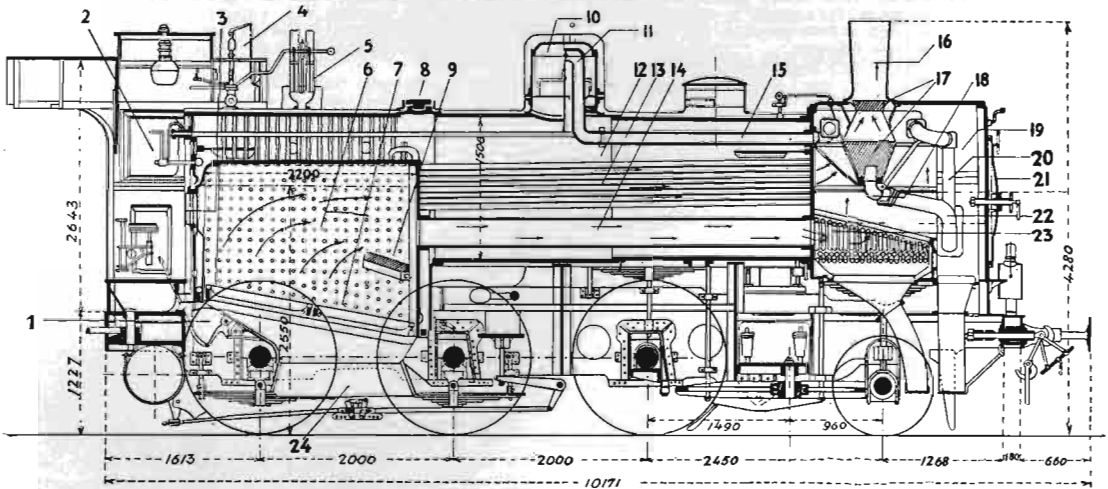
На сл.: 1. Механизам за отварање пепеоника. — 2. Полуа од регулатора. — 3. Ложишна врата. — 4. Парна звиждаљка. — 5. Вентил сигурности. — 6. Ложиште. — 7. Решетка. — 8. Отвор за чишћење. — 9. Ложишни свод. — 10. Скупљач паре. — 11. Регулатор. — 12. Котао. — 13. Грејне цев. — 14. Пламена цев. — 15. Паровод за прегрејач. — 16. Димњак. — 17. Варничара. — 18. Конус ексаустора. — 19. Димњача. — 20. Паровод за цилиндар. — 21. Врата на димњачи. — 22. Излазни паровод из цилиндра. — 23. Прегрејач. — 24. Пепеоник.
